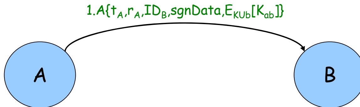
圖 4-3 單向認證
