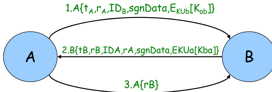
圖 4-6 三向認證
