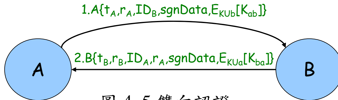
圖 4-5 雙向認證
